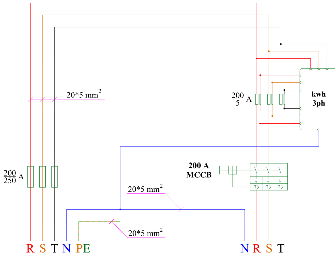
شکل ۳: دیاگرام تک خطی تابلوی تک کنتوری بارانی ۲۰۰ آمپری
