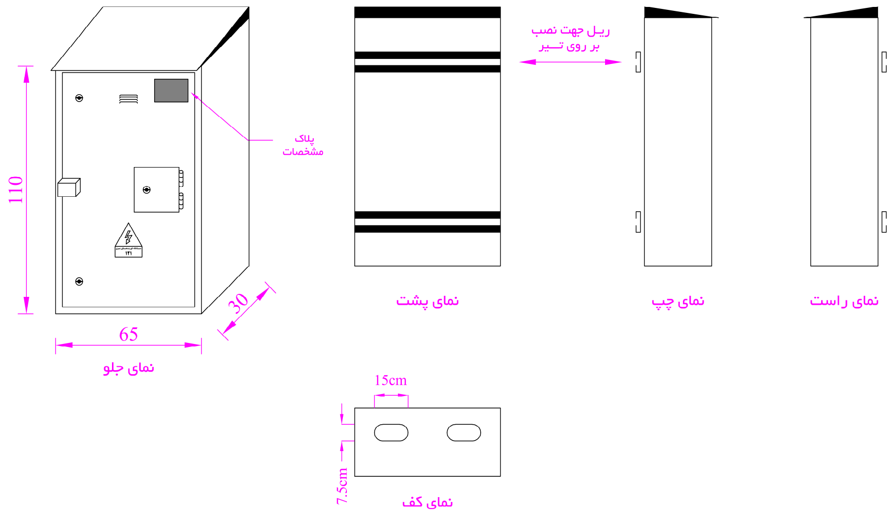
شکل ۱: نمای خارجی تابلوی تک‌کنتوری بارانی ۲۰۰ آمپری
