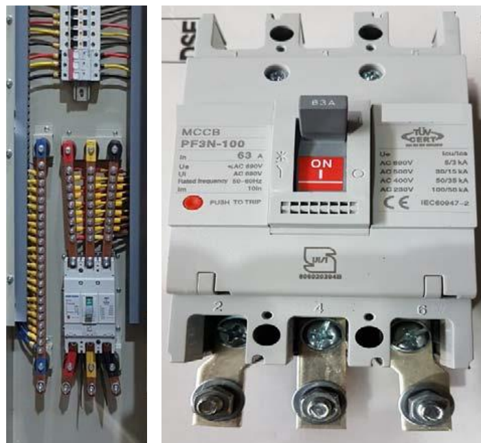
شکل ۳: الف) شینه‌های فابریک ب) شینه‌های کمکی کلید اتوماتیک
