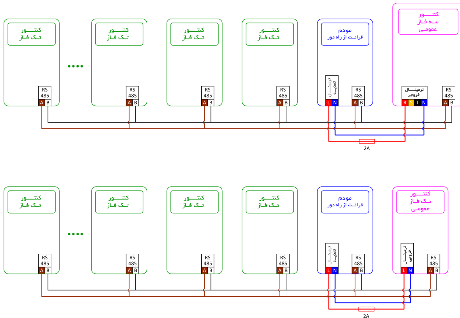
شکل ۹: نحوه سیم‌بندی مودم و کنتورهای هوشمند
